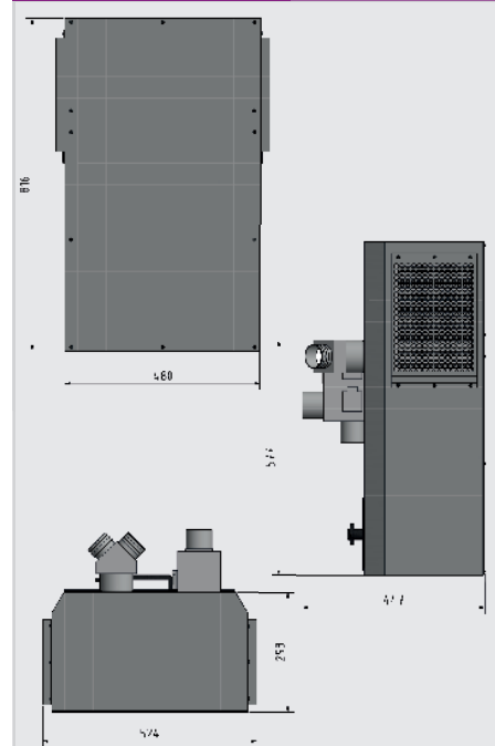
Gaveta de limalhas
