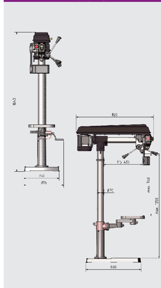
Dimensões RB 8S
