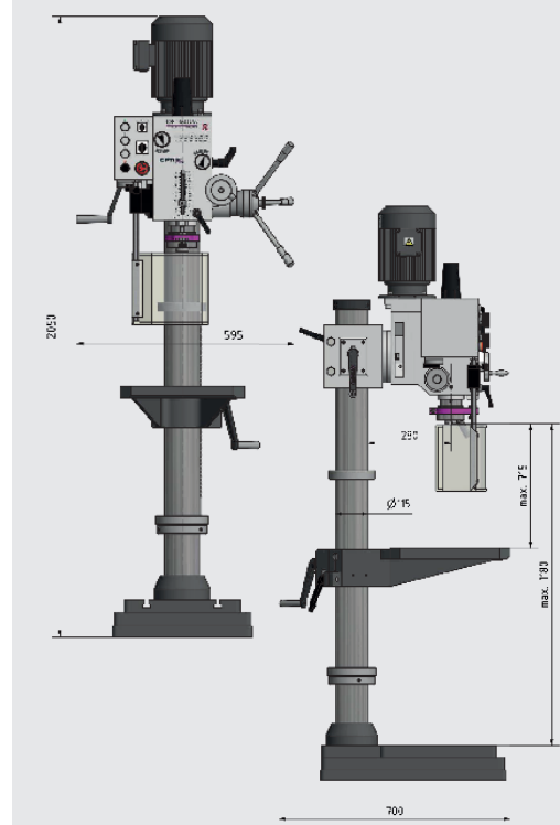
Dimensões DH 40GP
