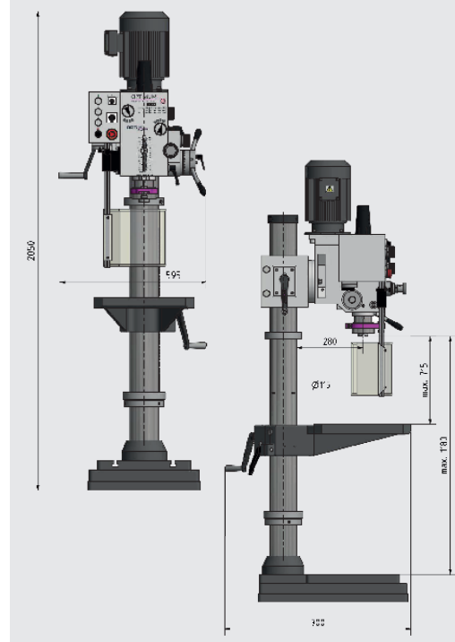
Dimensões DH 40GP
