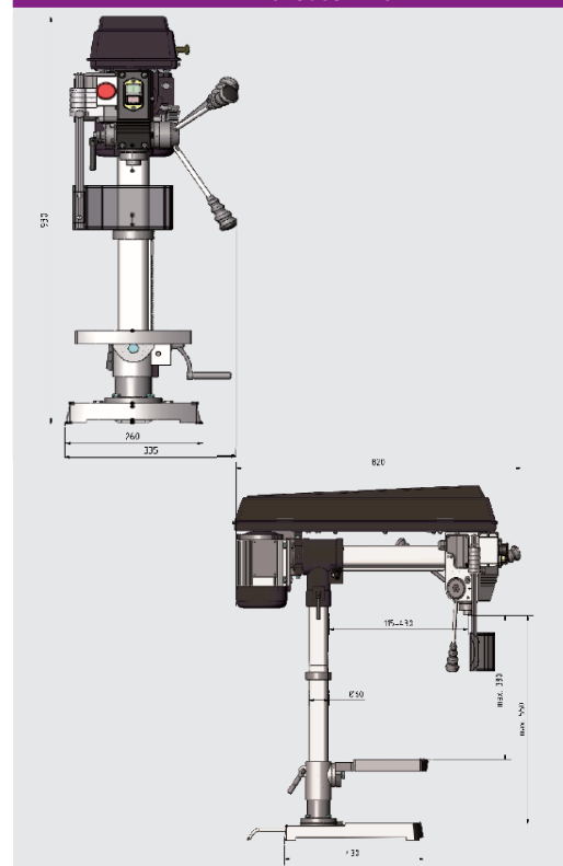
Dimensões RB 6T
