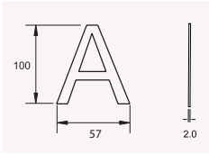
Dimensões / Dimensions
