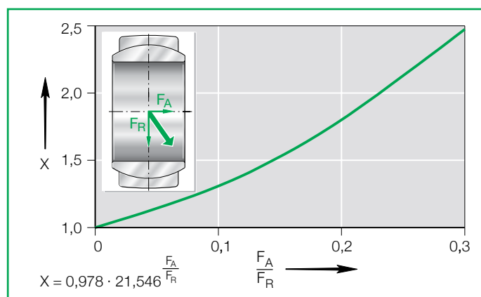
Snodi sferici radiali - carico combinato
