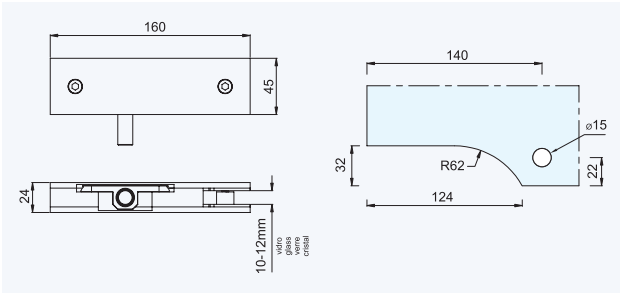
Pivot inferior Bottom pivot Pivot inférieur Pivot inferior
