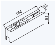
Opção posição do furo Pivot hole option
