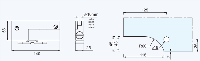
Pivot Superior Top pivot Pivot Supérieur Pivot Superior
