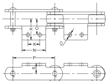
A-2 attacchi A-2 Attachment
