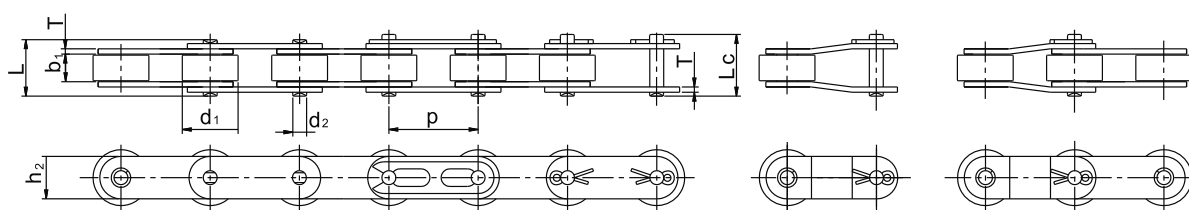
Rullo Maggiorato / Large Roller Type
