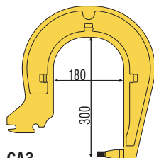
CA3 ARM + ELECTRODE L=300 mm - 803171
