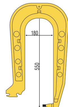
CA4 ARM + ELECTRODE L=550 mm - 803172
