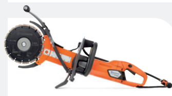
ELÉCTRICO HUSQVARNA K 4000 CUT-N-BREAK 230/120/110 V, 2700/1800/2200 W, 8,9 kg, tamaño de disco 230 mm, profundidad de corte 400 mm.
