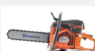
GASOLINA HUSQVARNA K 970 CHAIN 94 cc, 4,8 kW, 9,7 kg, tamaño de barra 350 mm, profundidad de corte 400 mm.
