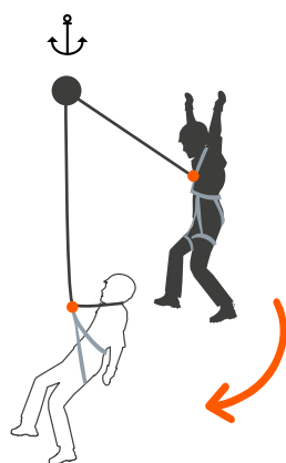
FATOR DE QUEDA 0
