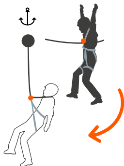
FATOR DE QUEDA 1
